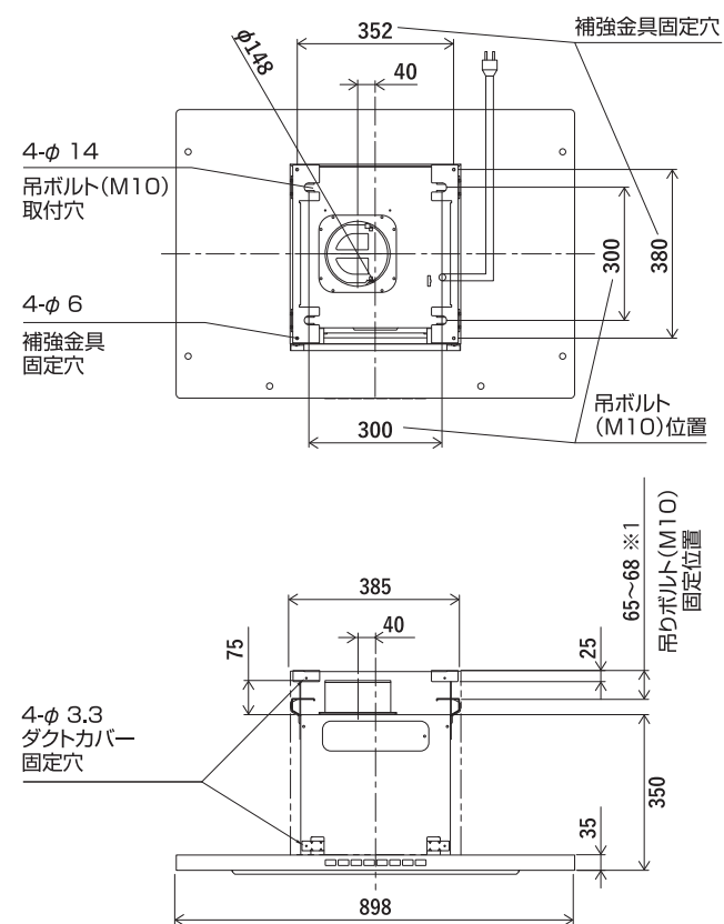
詳細図面(取付け高さ450mm)
