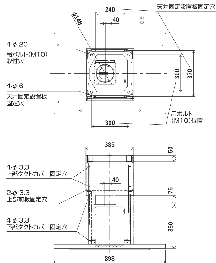
詳細図面(取付け高さ500~750/750~1000mm)
