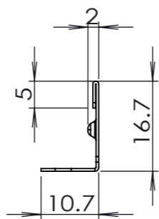
詳細図 A スケール 1:1
