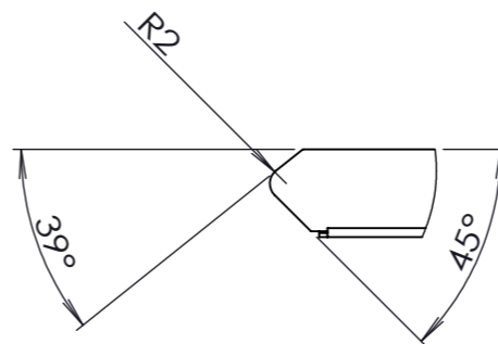
詳細図 B スケール 1:1
